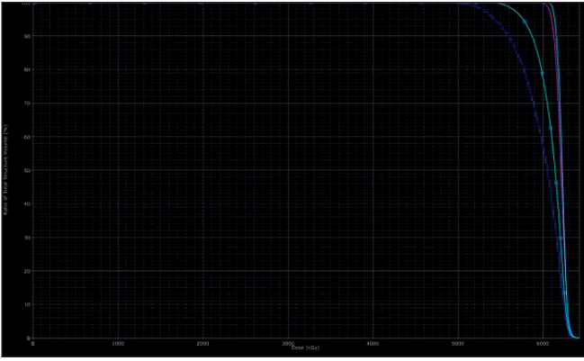
Resim. Radyoterapi DVH görüntüsü
