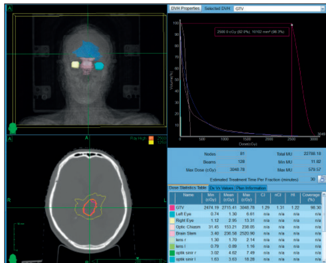
Resim. Doz volum eğrisi
