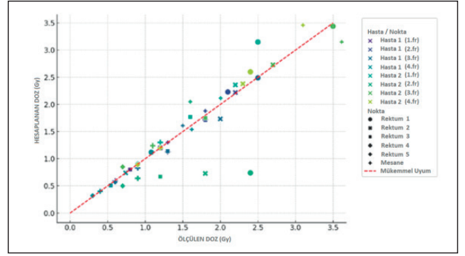
Grafik 2. Ölçülen ve Hesaplanan Mesane ve Rektum Dozlarının Dağılım Grafiği
