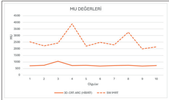
Resim. 3D-CRT-ARC ve SW-IMRT planlarında MU değerlerinin karşılaştırılması
