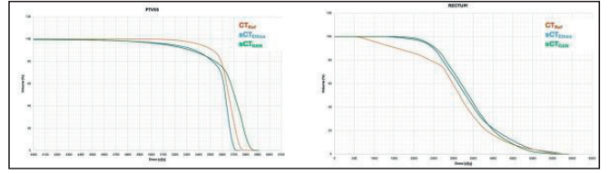
Resim 2. PTV55Gy ve rektum için Referans CTRef, sCTEthos ve sCTGAN 'lara göre hesaplatılmış DVH değerleri.
