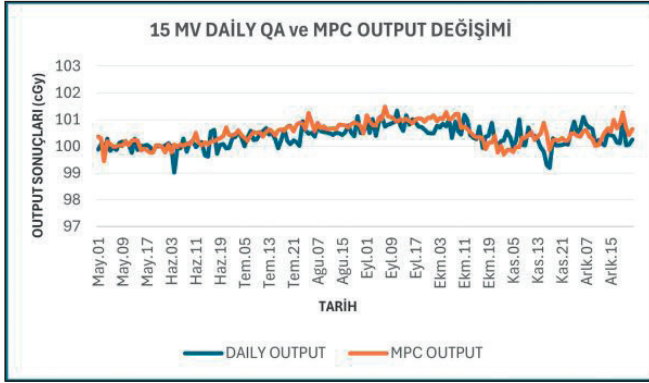
Resim. 15 MV Foton Enerjisi için Output Değişim Grafiği
