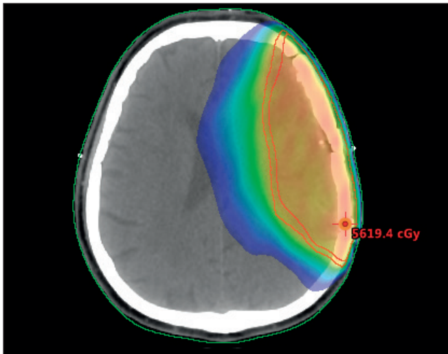
Resim 2. RPDR planı doz dağılımı, %50 izodoz
