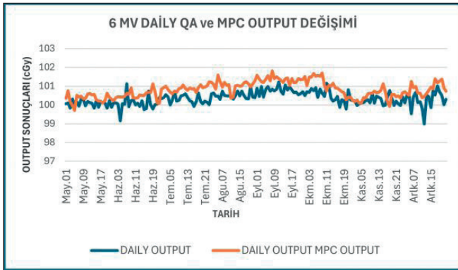
Resim. 6 MV Foton Enerjisi için Output Değişim Grafiği
