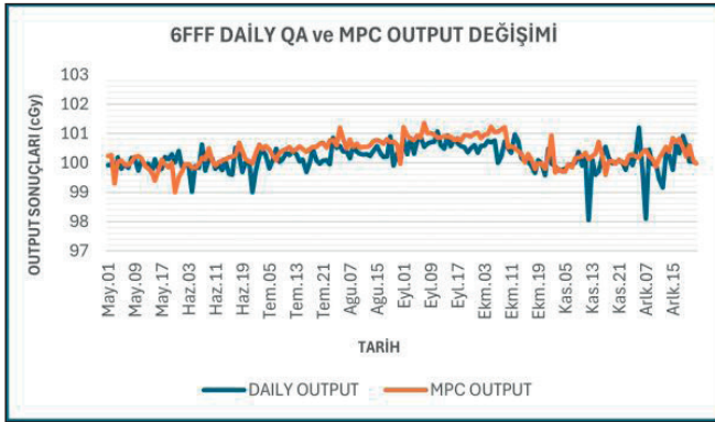
Resim. 6-FFF Foton Enerjisi için Output Değişim Grafiği
