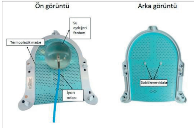
Resim 1. HSQA ölçümlerinde kullanılan küresel fantom ve iyon odası ile fantomun termoplastik maske ile sabitlenmesi.
