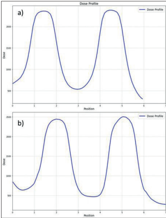
Resim 3. Lattice terapisi için doruk-vadi doz dağılımını gösteren doz profilleri. (a) 134 cc büyüklüğündeki bir GTV için iki lattice noktası arasındaki doz profilini, (b) ise 427 cc'lik daha büyük bir GTV için doz profilini göstermektedir.
