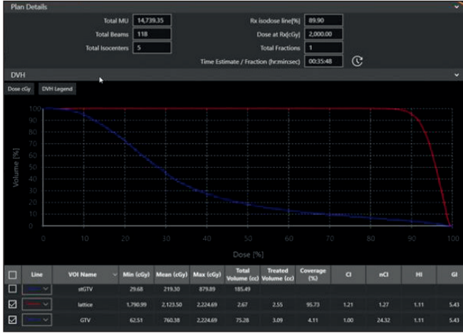
Resim 2. 75 cc büyüklüğündeki bir GTV için detaylı tedavi planı özeti sunmaktadır.
