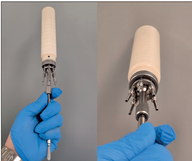
Resim 2. Yedi kanallı CT/MR uyumlu Miami Silindir Aplikatörü.
