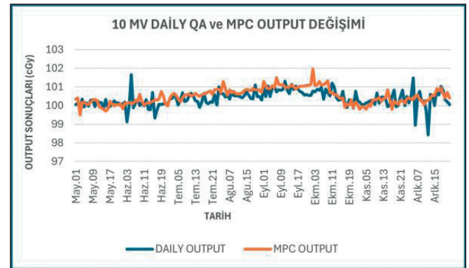
Resim 10. 10 MV Foton Enerjisi için Output Değişim Grafiği
